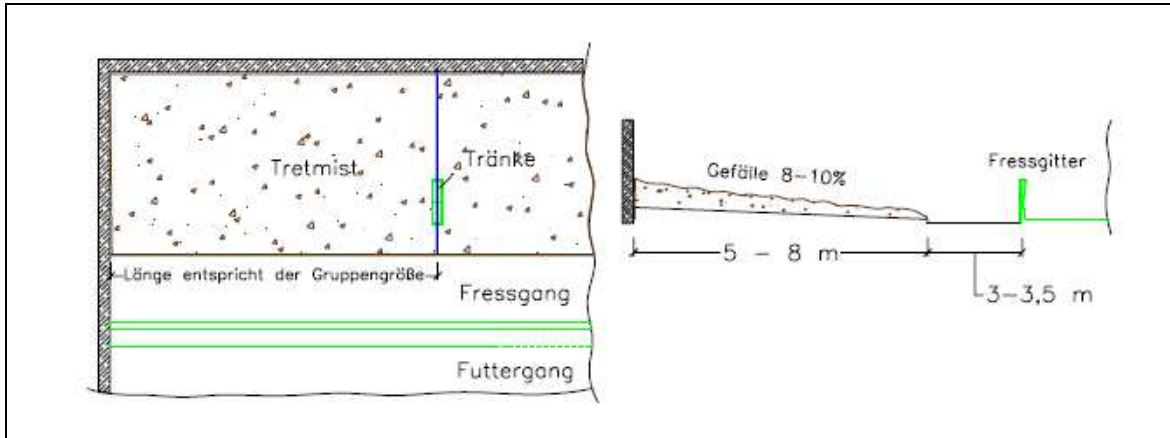
Abb. 7.4: Schema eines Tretmiststalls, hier verwendet in der Haltung von Färsen
