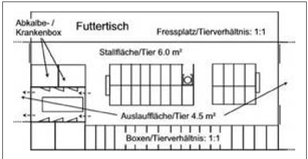
Abb. 7.2: Boxenlaufstall zur Haltung von Milchkühen, gemäß den Anforderungen der EG-Öko-Verordnung
